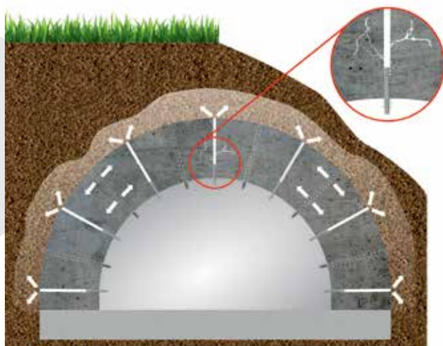
Возможность инъектирования в конструкцию и за конструкцию
