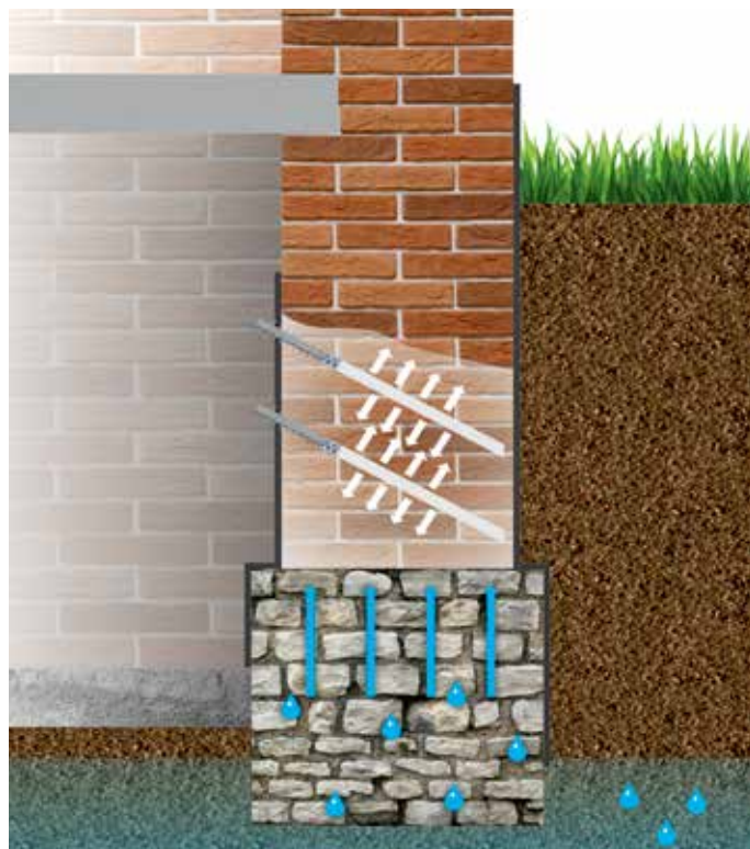
Отсечная гидроизоляция бутового фундамента
