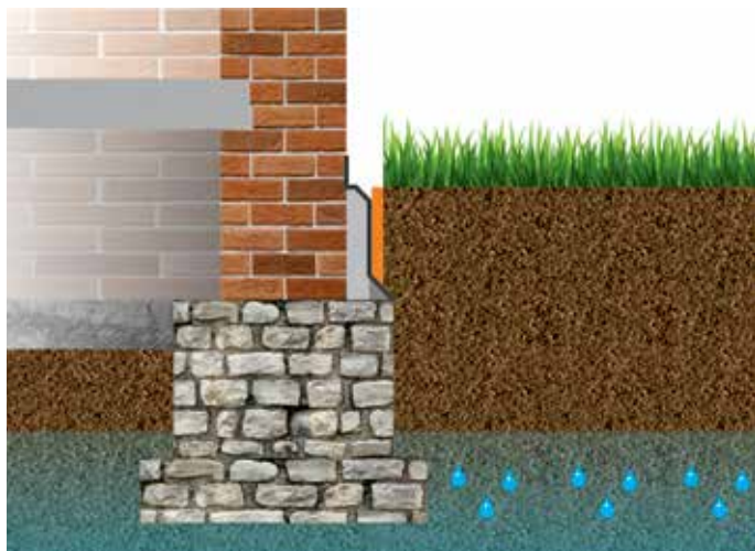
Гидроизоляция конструкции снаружи
