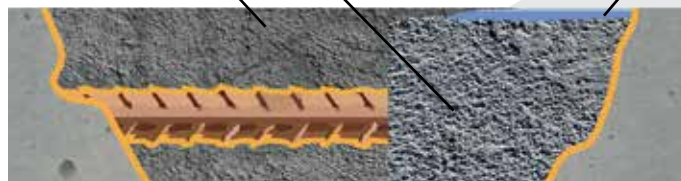
Послойный ремонт дефекта бетонной конструкции
