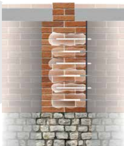
Усиление кирпичной стены
